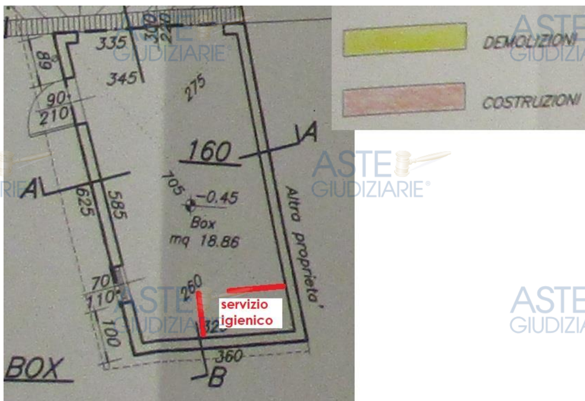
Estratto tavola 4 – stato di progetto – DIA 356/2011
